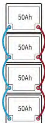
Паралельне підключення 12В (12,8В) 200Ah
