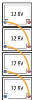
Послідовне підключення 48В (51,2В) 50Ah
